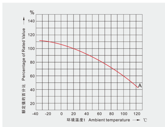
環境溫度--承載能力曲線
